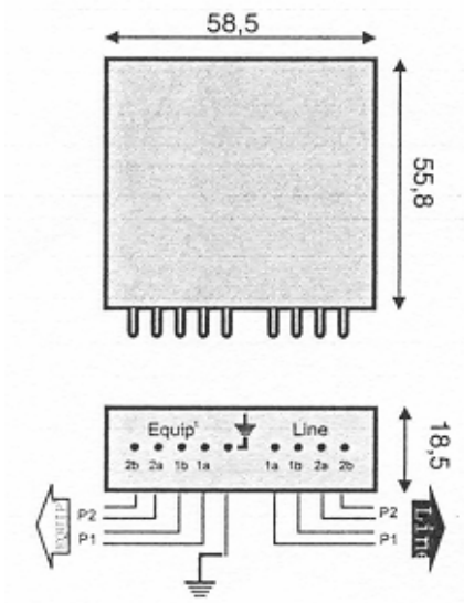
2 Pair 48V Module
