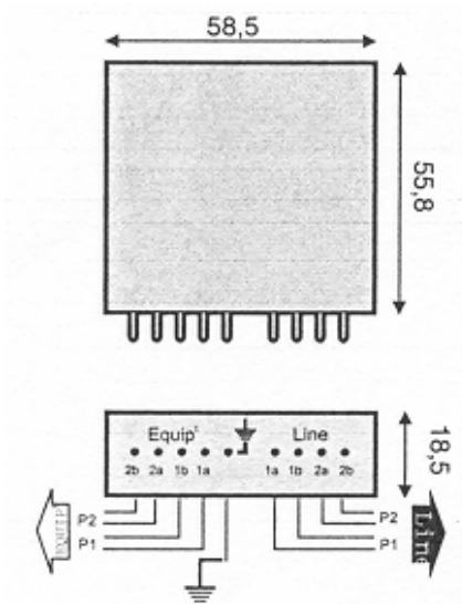
2 Pair 12V Module
