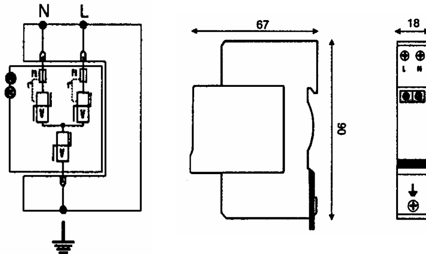
D.I.N - 120 Volt AC Protection Module
